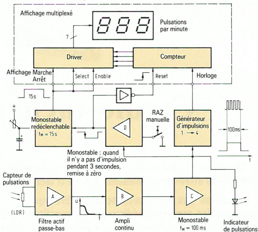
Fig. 1. – Schéma synoptique de l'appareil.
