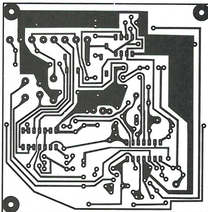
Fig. 5. — Le circuit imprimé principal.
