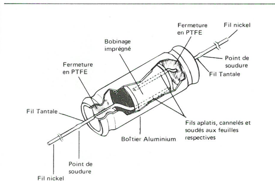
Fig. 1 – Structure d'un condensateur tantale-feuille.
