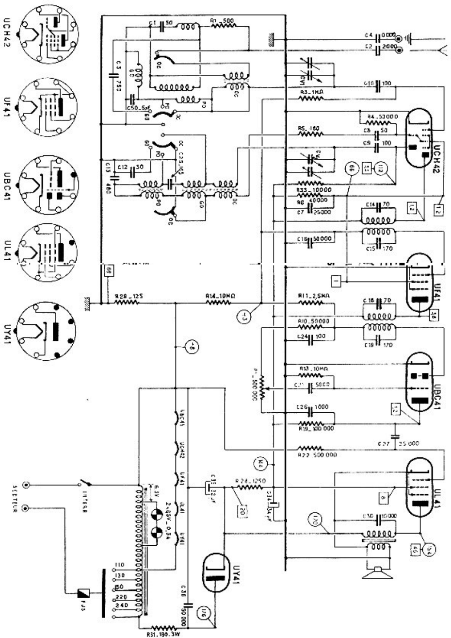
Schéma général du récepteur D925.
