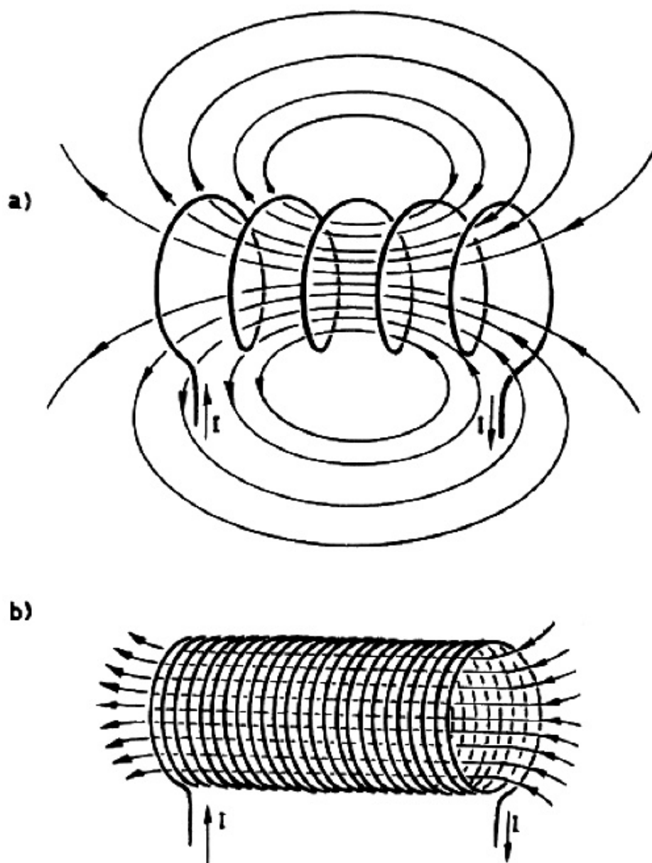
BOBINES ET LEUR CHAMP MAGNETIQUE
